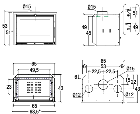
Model: IL 65/49 *Dimensioni con profil./Dimensions with trims.
