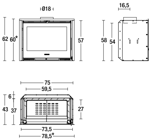
Model: IL 75/58 *Dimensioni con profili./Dimensions with trims.
