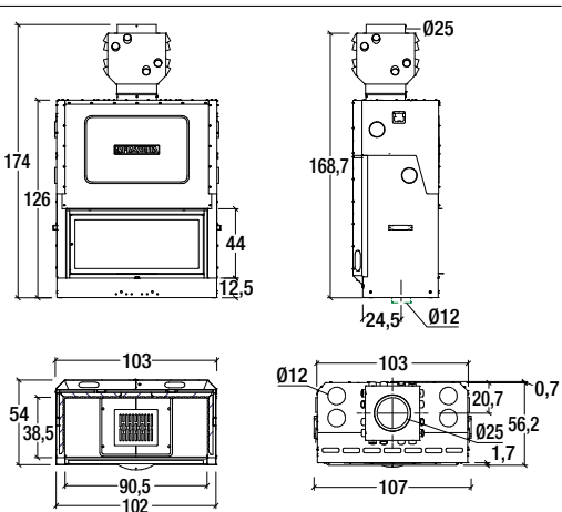
Model: MA 263 SL PLUS
