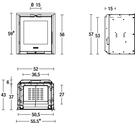
Model: IL 52/57 *Dimensioni con profil./Dimensions with trims.
