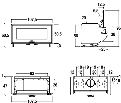
Model: MC 105/48 BL
