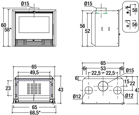
Model: IL 65/56 V
