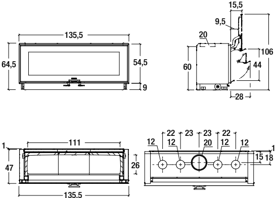
Model: MC 133/52 BL
