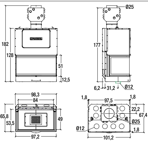
Model: MA 271 SL PLUS
