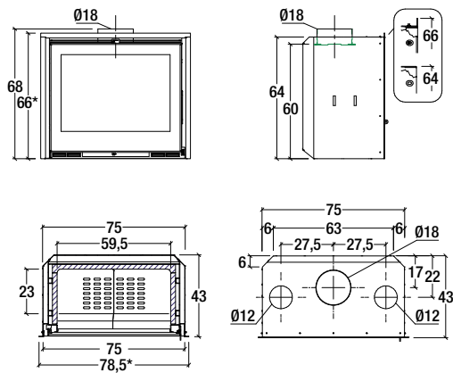
Model: IL 75/64 *Dimensioni con profili./Dimensions with trims.
