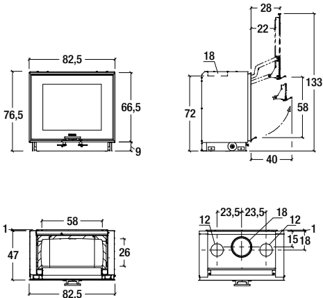
Model: MC 80/64 BL
