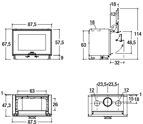
Model: MC 85/55 BL
