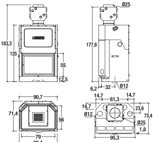
Model: MA 261 SL PLUS
