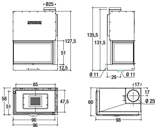
Model: MA 283 DX SL - MA 283 SX SL
