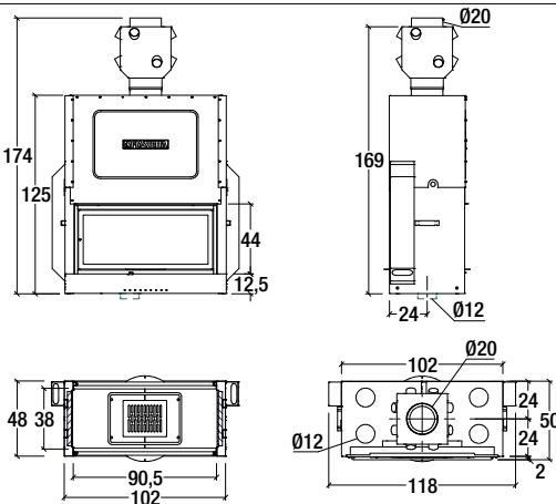
Model: MA 263 B SL PLUS
