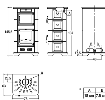
Model: E900 M
