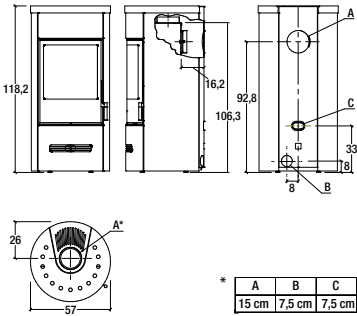
Model: E129 M
