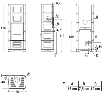
Model: E928 C-M
