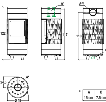
Model: CIRCLE BCS
