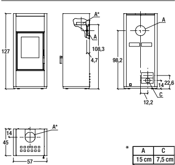
Model: E128 BCS
