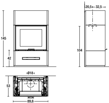
Model: BERN A
