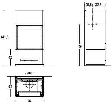
Model: BERN A
