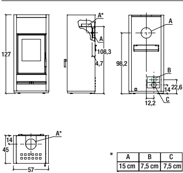
Model: E128 BCS
