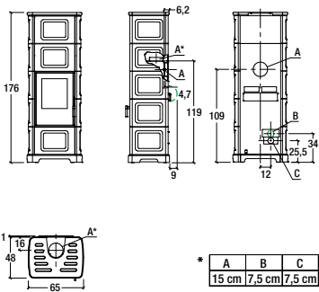
Model: E928 C-M BCS
