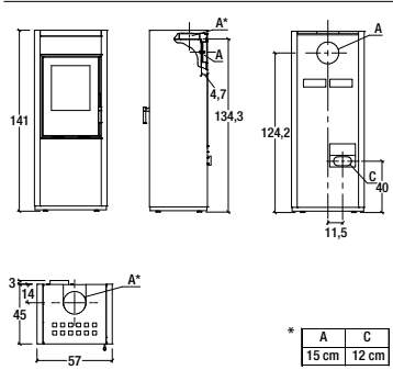
Model: E128 A
